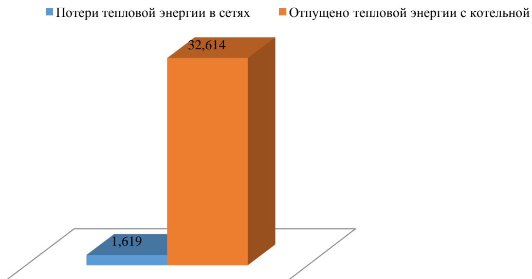
Рисунок 1.4. Величина потерь согласно первому сценарному плану
